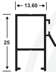
2623 ENGANCHE
