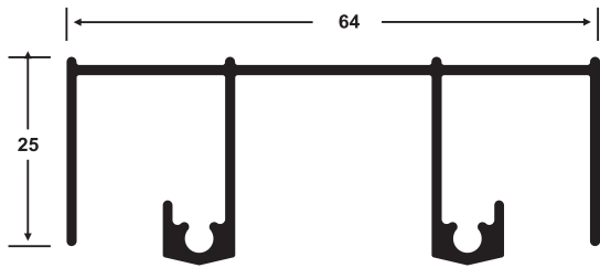
2801 Doble Riel Superior
