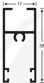
2004 CABEZAL
