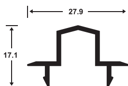
62506 ADAPTADOR DE HOJA
