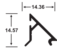
3503 Junquillo
