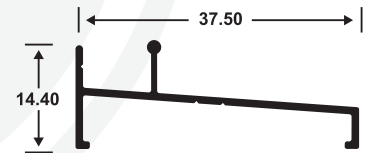
2627 RIEL INFERIOR
