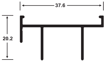
2920 Doble Riel Superior
