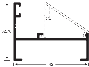
4209 MARCO
