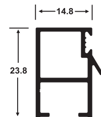
2923 Enganche
