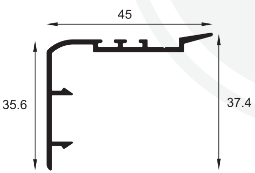
80506 ADAPTADOR DE HOJA
