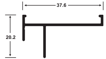
2926 Riel Superior
