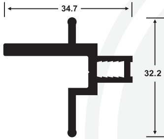
4504 Clip de sujeción horizontal
