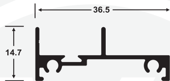
2928 Marco Móvil
