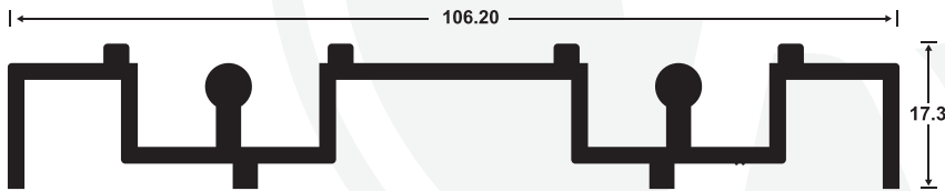
7010 Sillar
