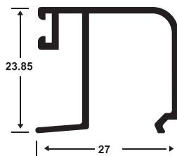
3608 JUNQUILLO 8MM
