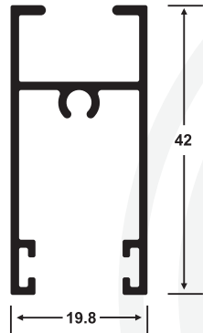
2804 Cabezal
