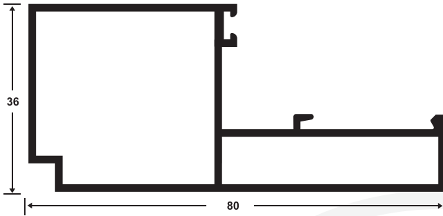
3601 MARCO LATERAL
