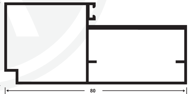
3613 MARCO LATERAL
