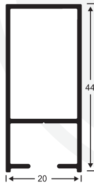
2010 PARANTE
