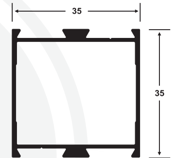
3508 Bastidor
