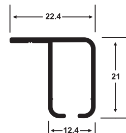
PERFIL CORTINERO
