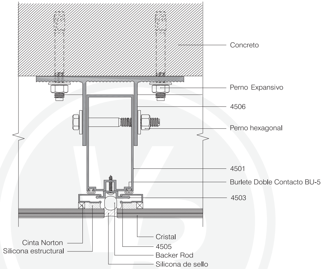
MURO CORTINA VISTA HORIZONTAL
