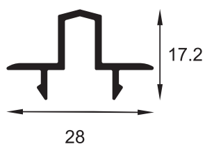
80506 ADAPTADOR DE HOJA
