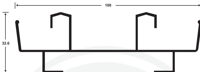
62701 MARCO DOBLE CORREDIZA
