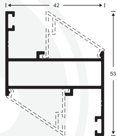
4202 MARCO NAVE
