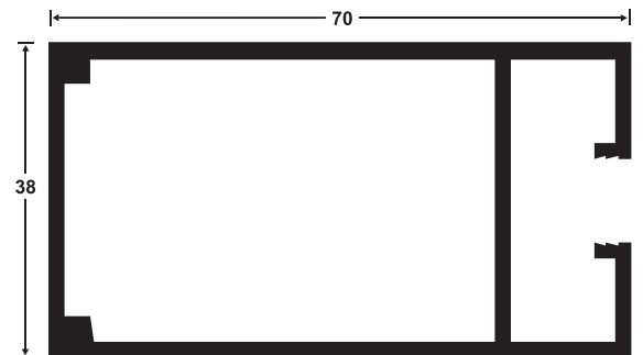
7040 Traslape
