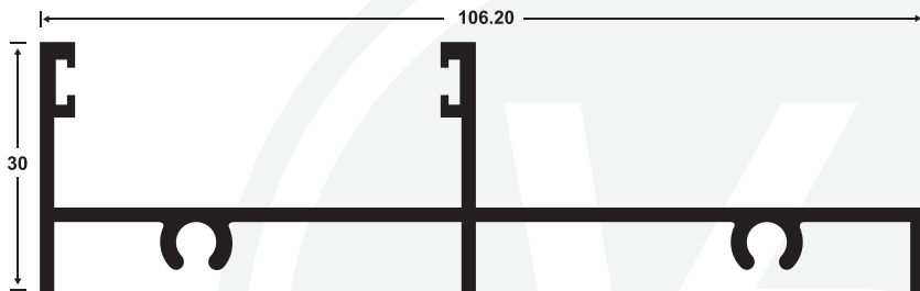
7020 Jamba
