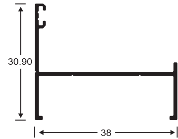
172 Marco
