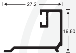
4206 JUNQUILLO P/INSULADO
