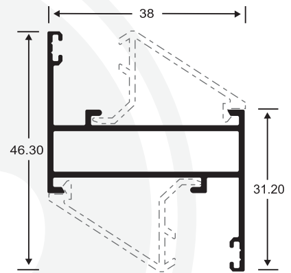
176 Marco Nave
