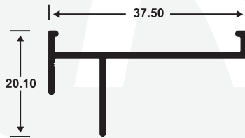
2626 RIEL SUPERIOR
