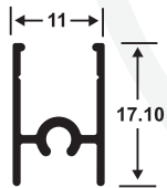
2625 HORIZONTAL FIJO
