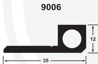
PERFIL P/PIC ZOCALO
