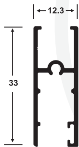
2924 Horizontal Móvil
