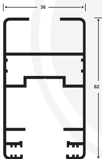
62703 MARCO DE HOJA
