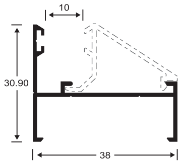
173 Marco
