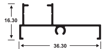
2629 MARCO FIJO
