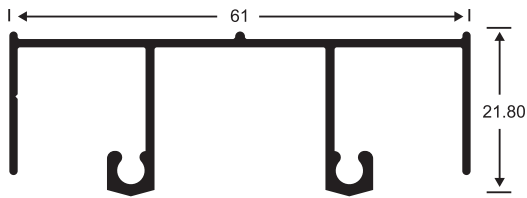
2001 DOBLE RIEL SUPERIOR
