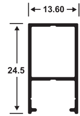
2622 PARANTE
